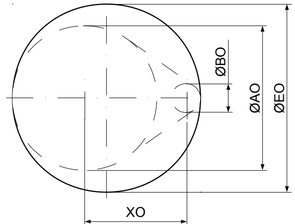
Einbauöffnung-Mindestmaße
